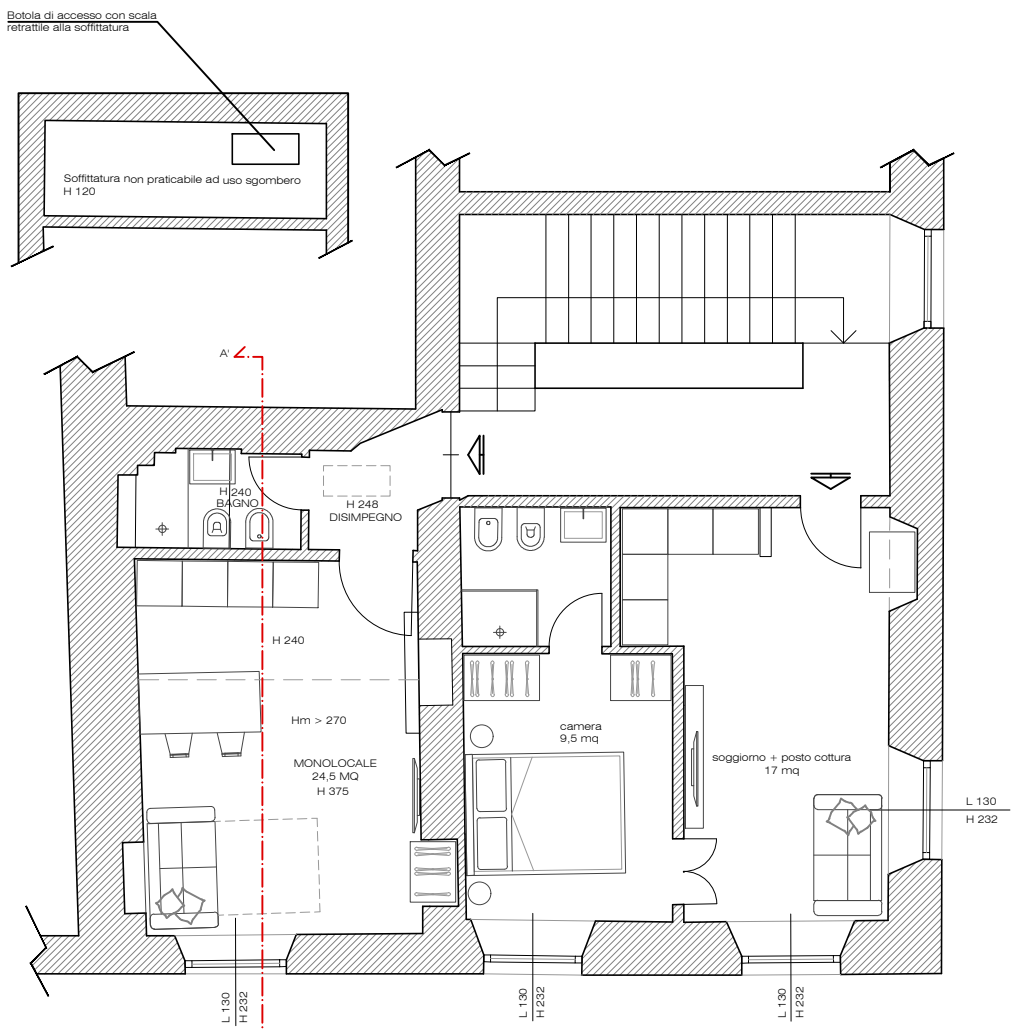
STATO di PROGETTO
