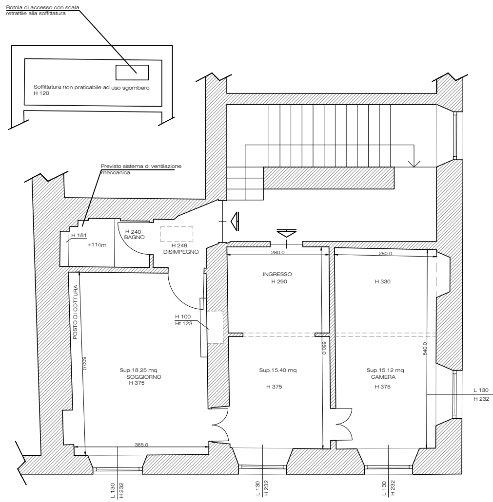
STATO di FATTO
