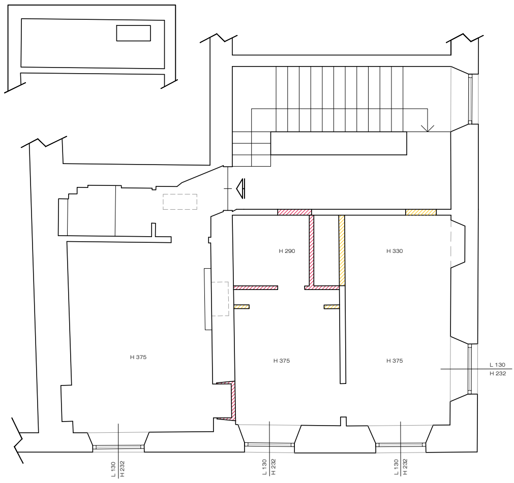
STATO di RAFFRONTO
